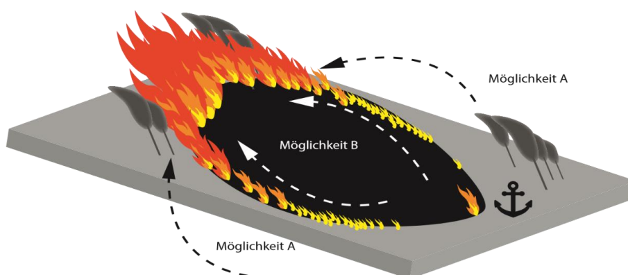
Abb. 6.13: Angriff aus dem Schwarzbereich über die Flanken [5]
